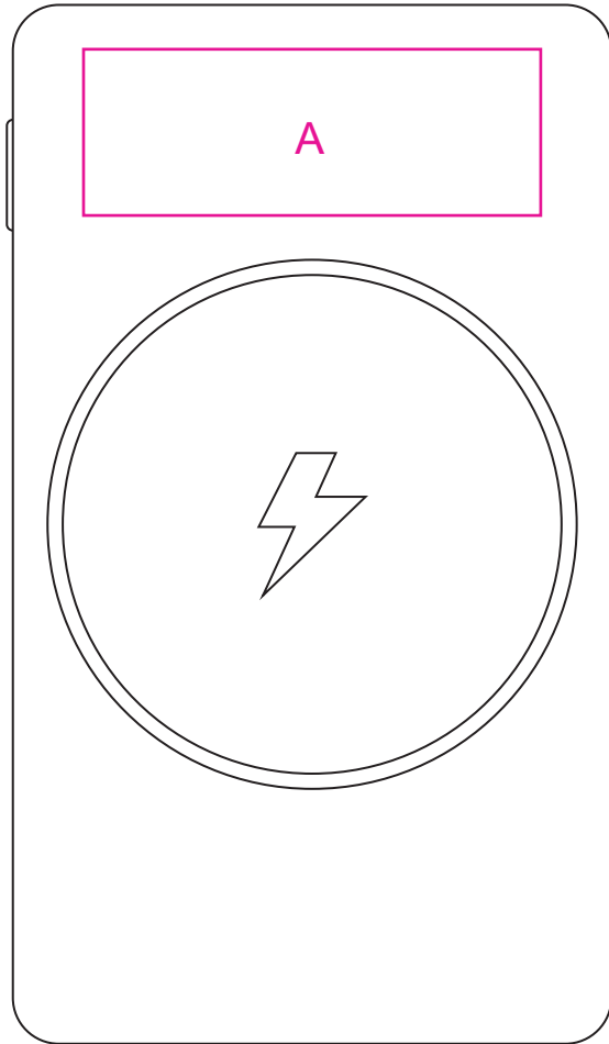
A: Engraving size: 55mm(w) x 20mm(h) Shown at 100% actual size
